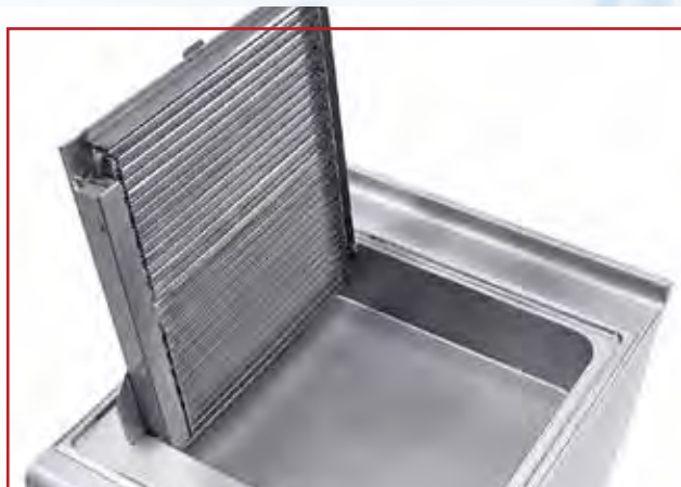
Nahtlose tiefgezogene Fettauffangwanne für einfache und sichere Reinigung
